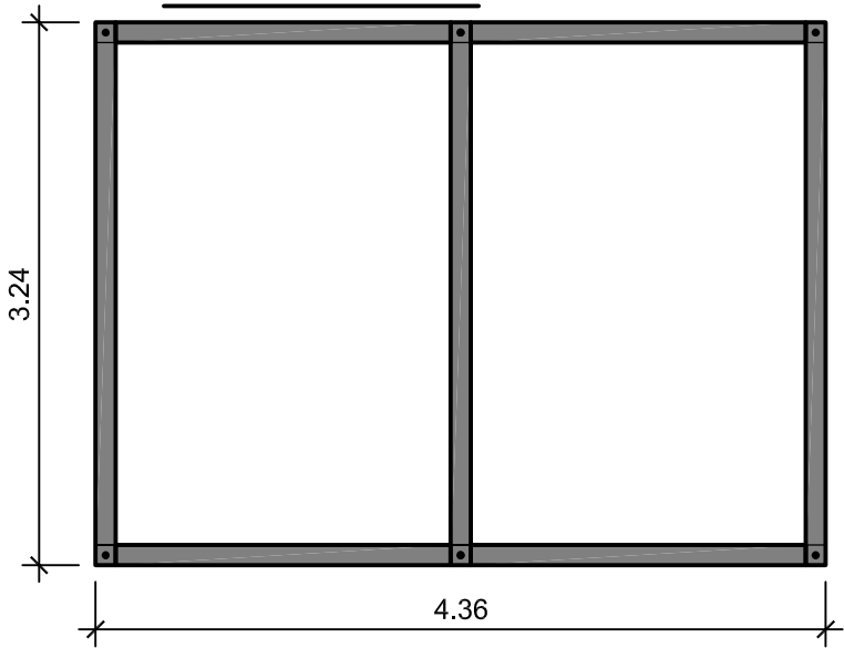
Grundriss 1:50
